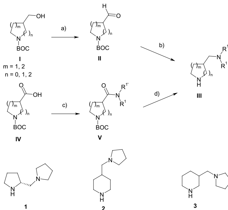
Scheme 1. (a) \text{DMSO} , (\text{COCl})_2 , \text{Et}_3\text{N} ; (b) (i) \text{HNR}^1 \text{R}^{1'} , \text{NaBH}(\text{OAc})_3 , \text{HOAc} (ii) \text{TFA} ; (c) \text{EDAC} , \text{DHOBT} , \text{Et}_3\text{N} ; (d) (i) \text{TFA} , (ii) \text{LiAlH}_4 .
